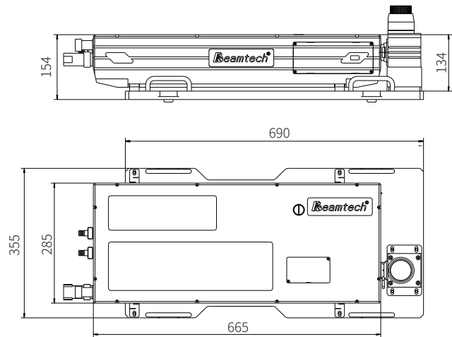
Vlite-532-E激光头
