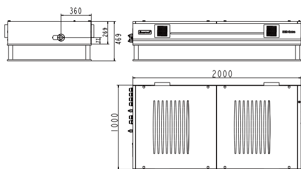
激光头 (供参考, 定制)
